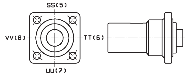
ÖLANSCHLUSS-U., HINTERSEITE.
