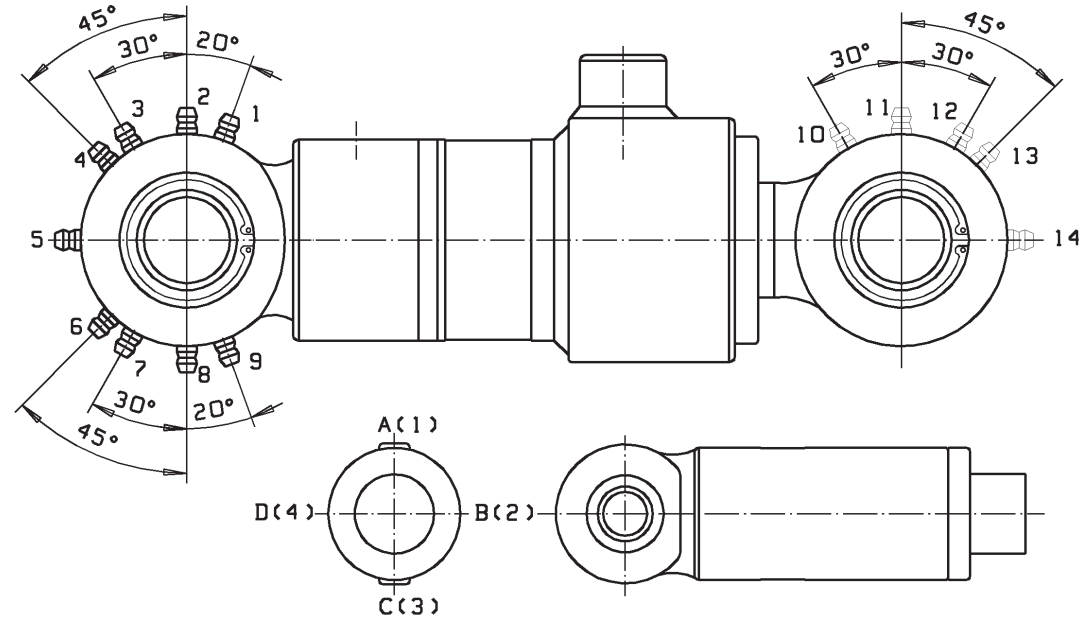
ÖLANSCHLUSS-U., VORDERSEITE.
