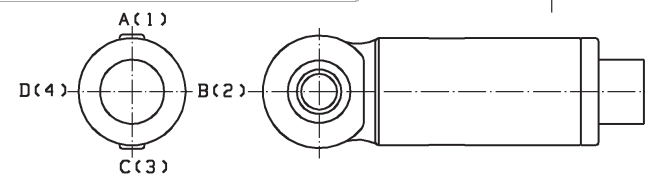
ÖLANSCHLUSS-U., VORDERSEITE.
