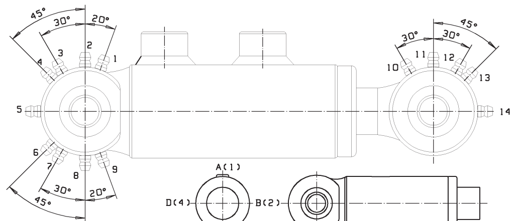
ÖLANSCHLUSS-U., VORDERSEITE.
