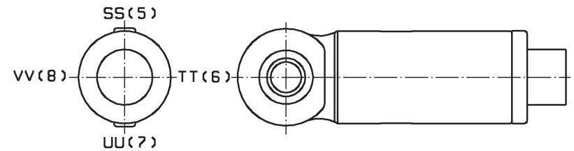
ÖLANSCHLUSS-U., HINTERSEITE.
