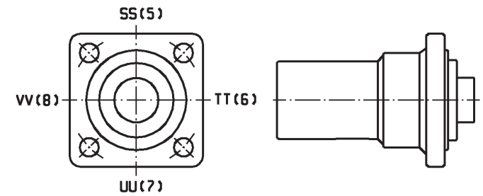
ÖLANSCHLUSS-U., HINTERSEITE.
