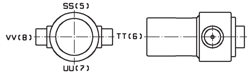
ÖLANSCHLUSS-U., HINTERSEITE.
