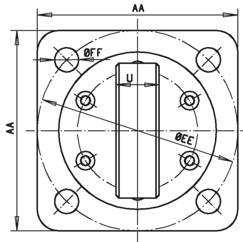
ÖLANSCHLUSS-U., VORDERSEITE.
