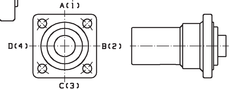
ÖLANSCHLUSS-U., VORDERSEITE.
