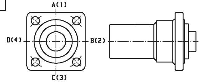
ÖLANSCHLUSS-U., VORDERSEITE.
