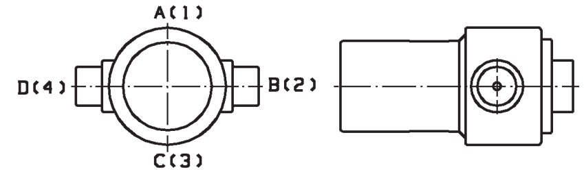
ÖLANSCHLUSS-U., VORDERSEITE.
