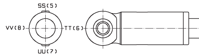
ÖLANSCHLUSS-U., HINTERSEITE.
